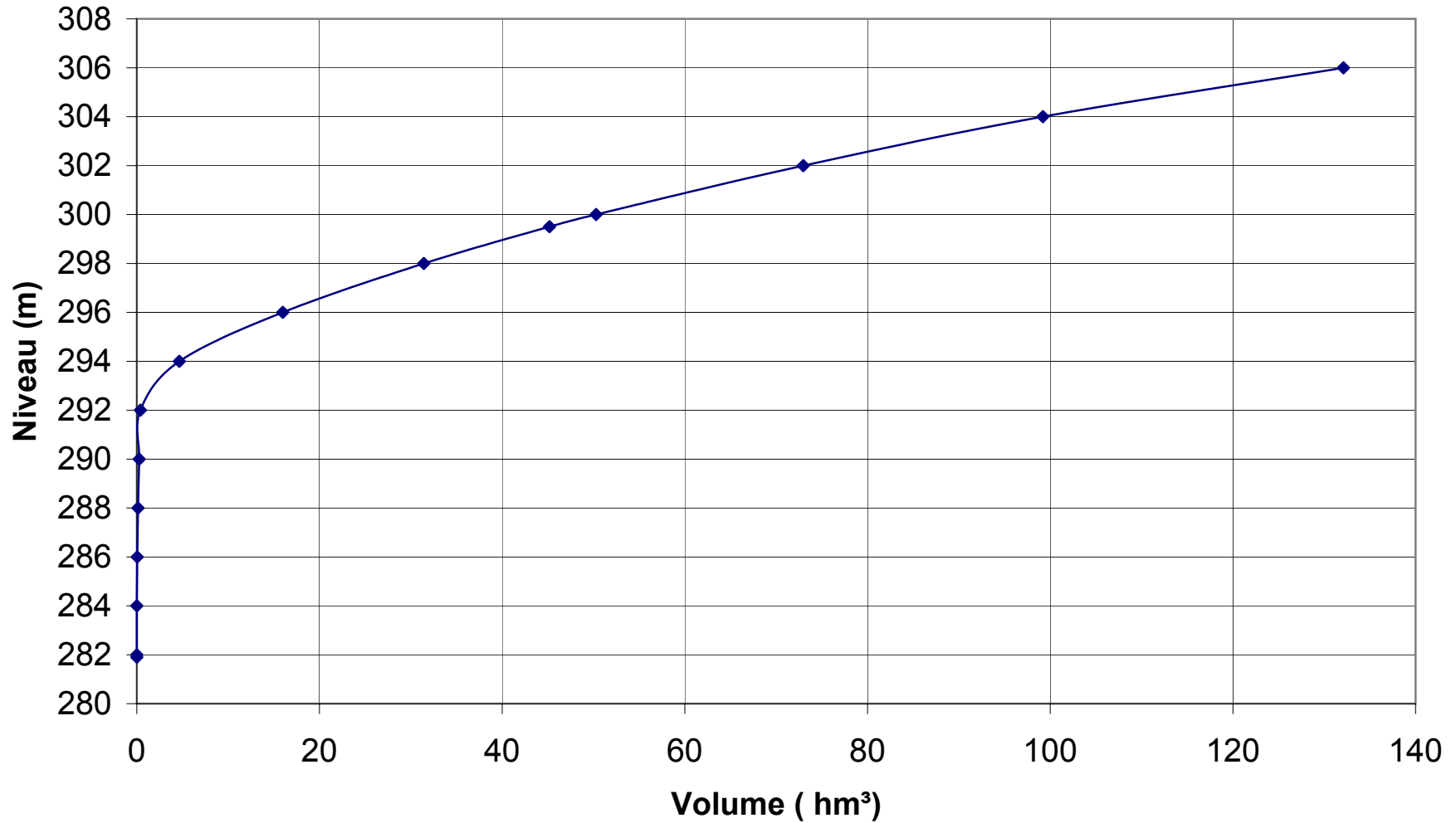
Figure 2.9 Courbe d'emménagement du bief d'amont de Rapides-des-Coeurs
