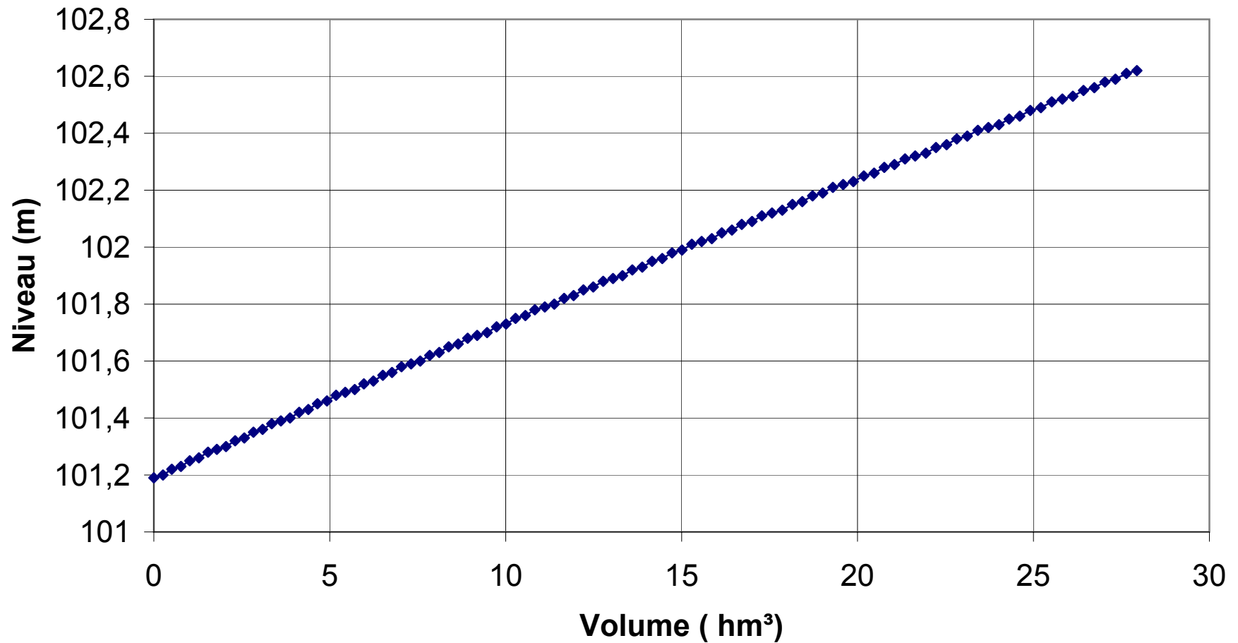
Figure 2.6 Courbe d'emmagasinement du bief d'amont de l'aménagement de Grand-Mère
