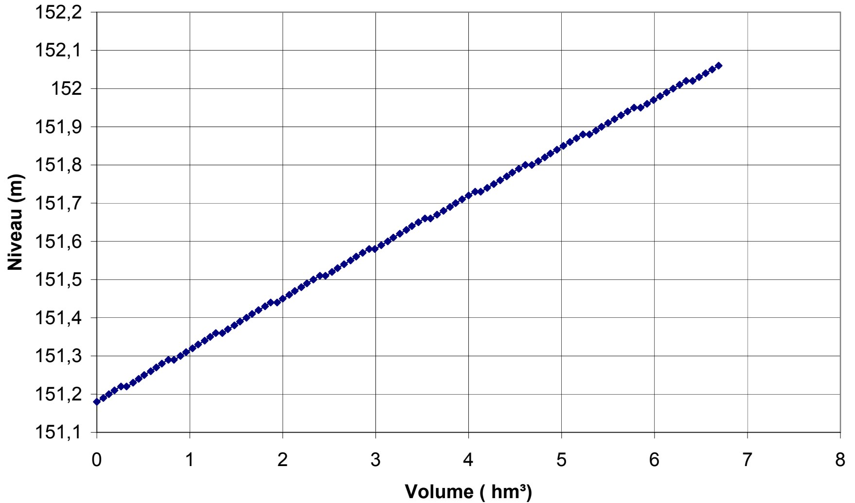
Figure 2.5 Courbe d'emménagement du bief d'amont de LaTuque
