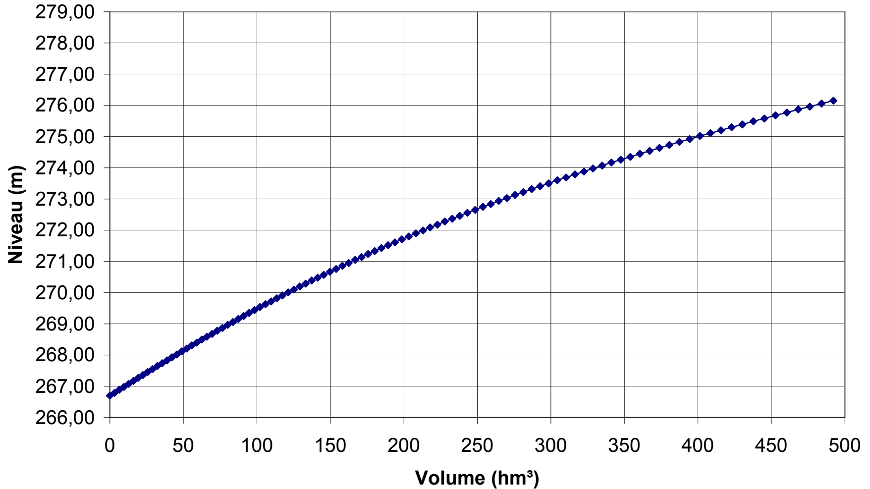
Figure 2.2 Courbe d'emménagement du réservoir Rapide-Blanc
