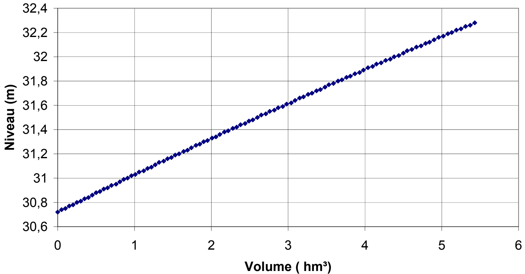
Figure 2.8 Coubre d'emmagasinement du bief d'amont de l'aménagement La Gabelle
