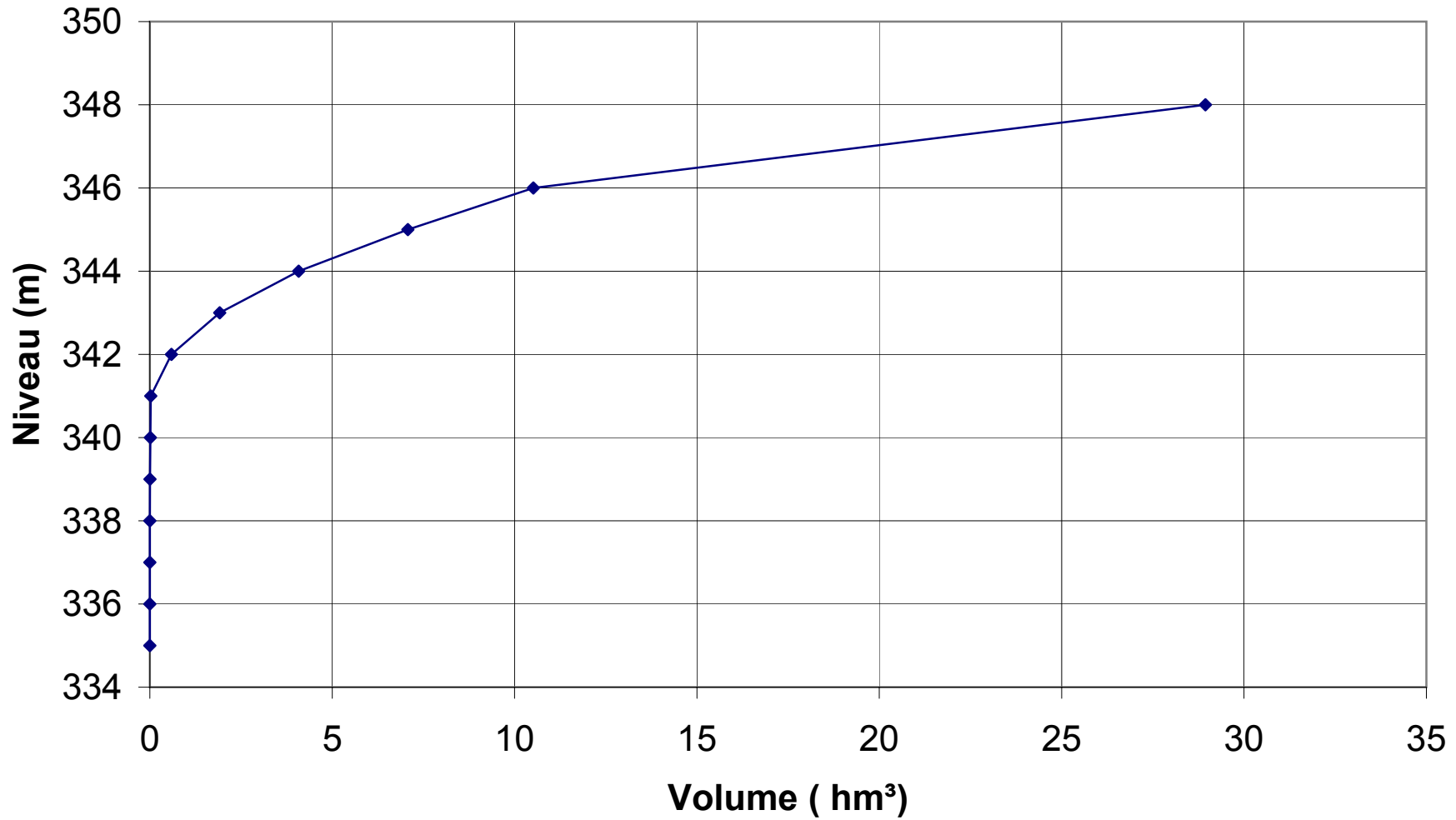
Figure 2.10 Courbe d'emmagasinement du bief d'amont de Chute-Allard
