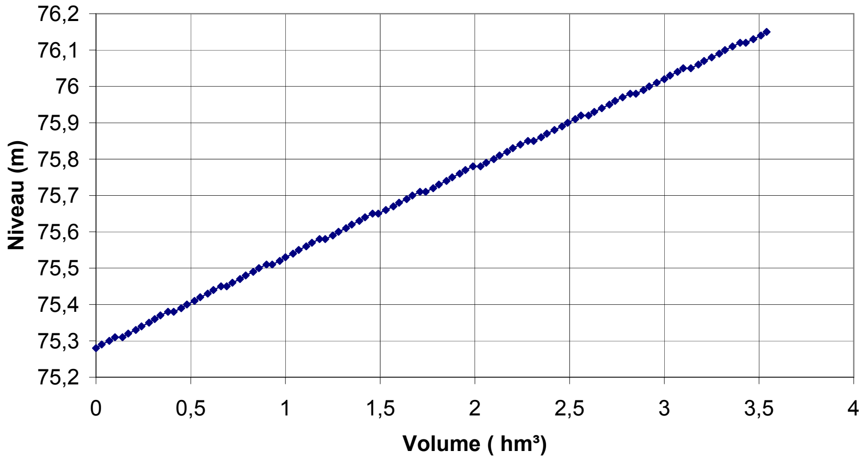
Figure 2.7 Courbe d'emmagasinement du bief d'amont de l'aménagement Shawinigan
