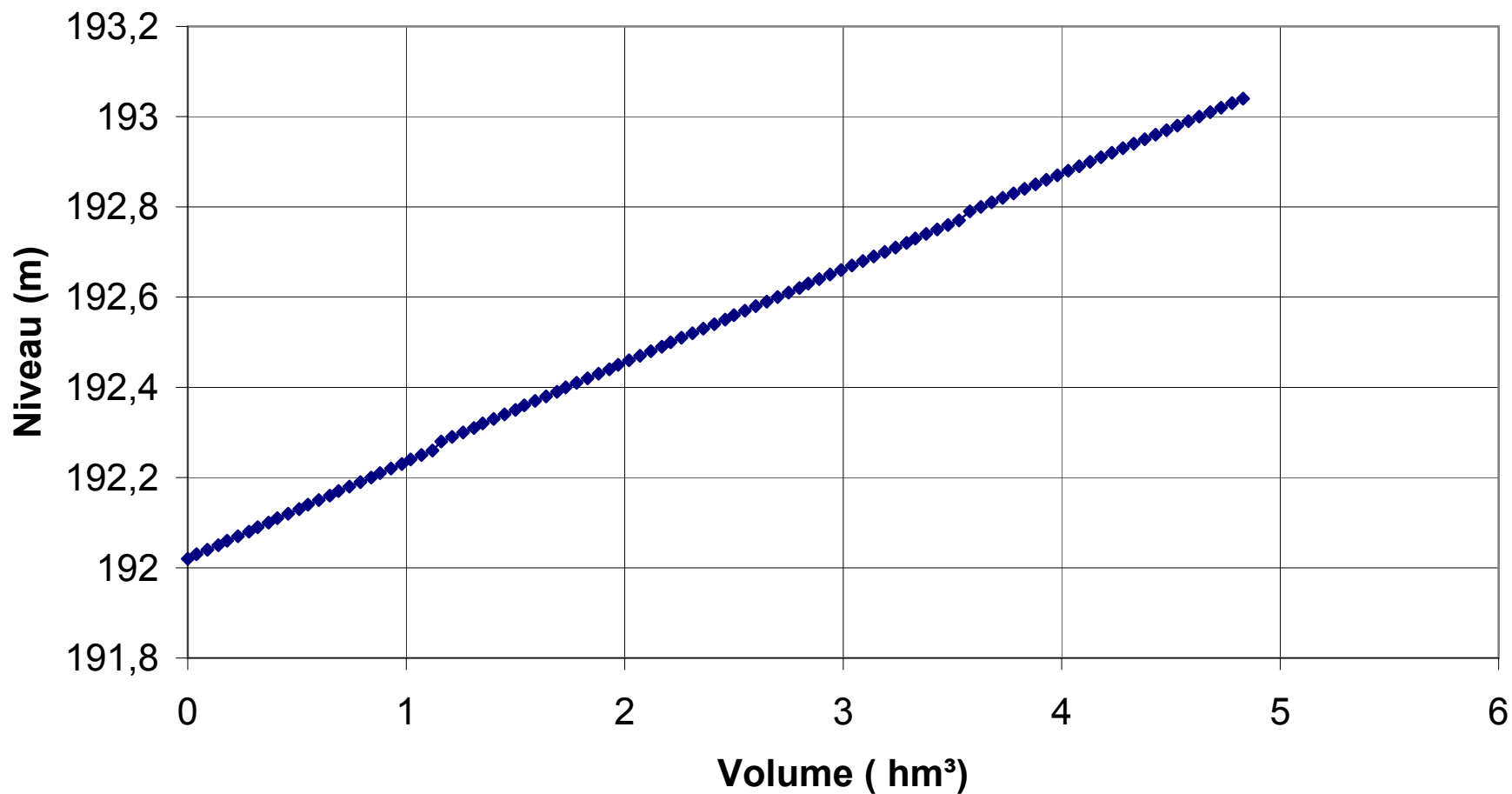
Figure 2.4 Courbe d'emmagasinement du bief d'amont de l'aménagement Beaumont
