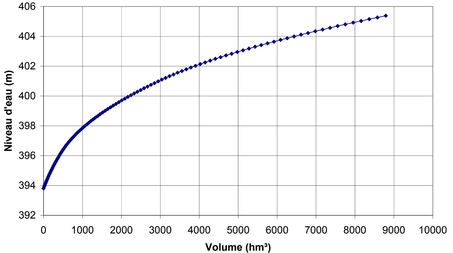
Figure 2.1 Courbe d'emmagasinement du barrage Gouin
